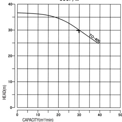
TO-400型 性能曲線図 600r/m
